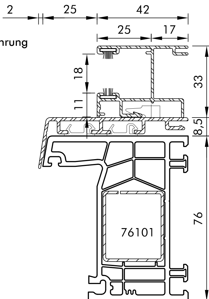
P 6180 Rolladenabrollprofil
