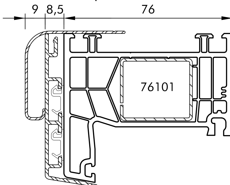
P 6180 Rolladenabrollprofil
