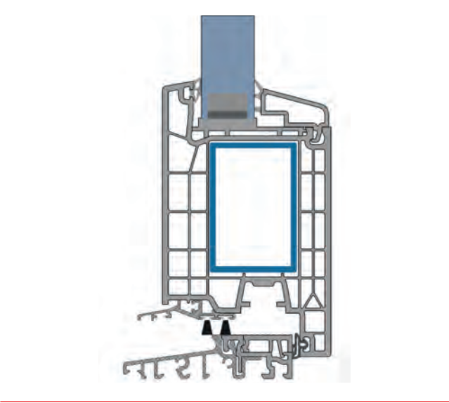
PROFILDISEIGN DER BASIC-BAUREIHE
