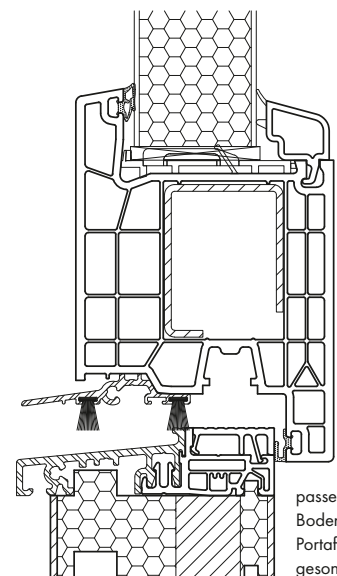
Profildesign der Basic-Baureihe
